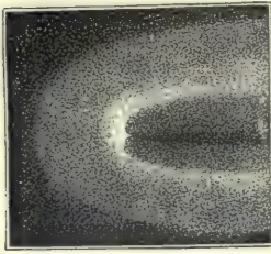
September 29. (Pepe.)
